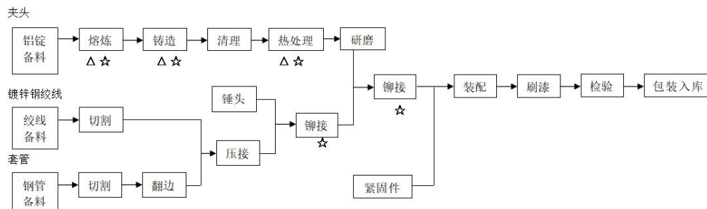
防振锤工艺流程图
